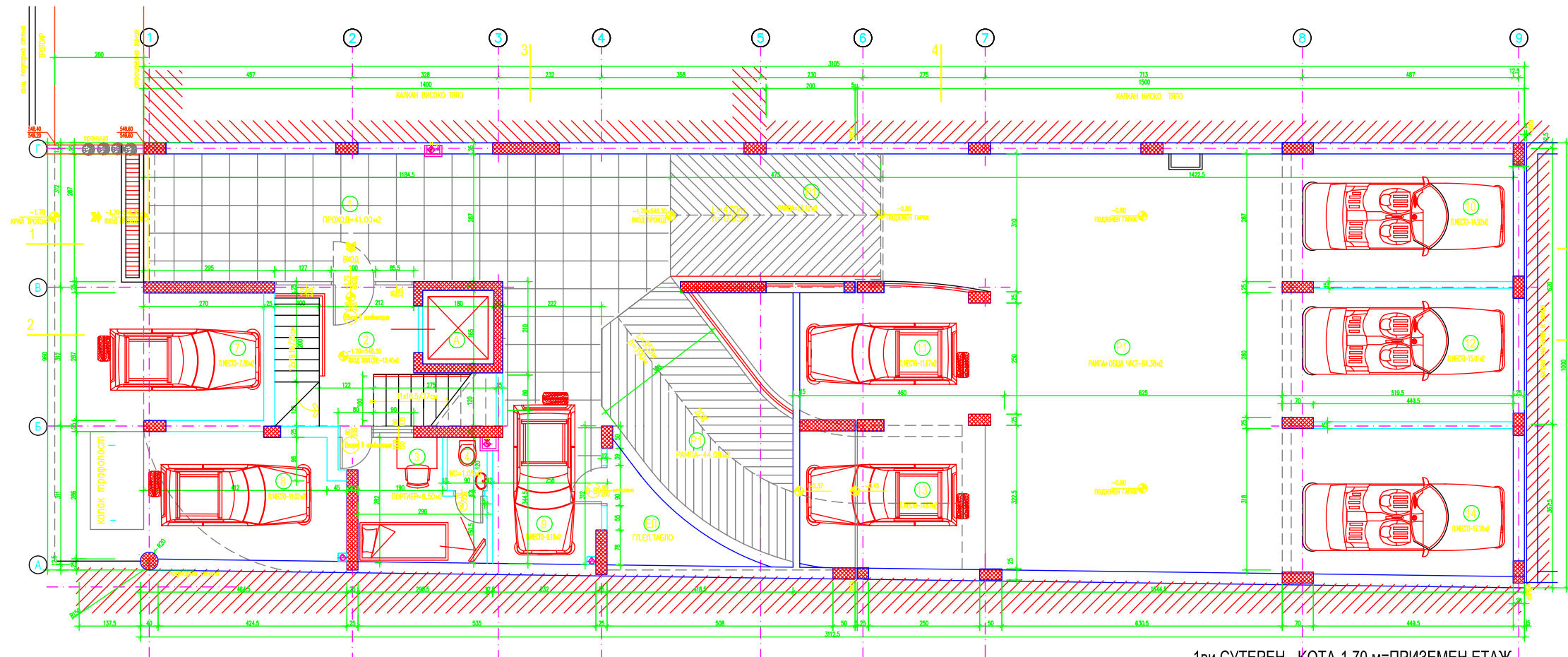
1ви СУТЕРЕН - КОТА-1.70 м=ПРИЗЕМЕН ЕТАЖ
